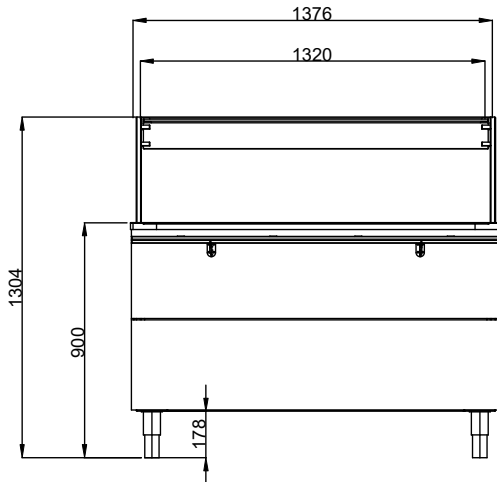
Alzado
